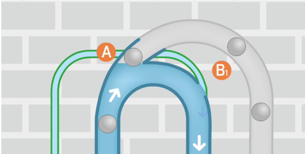
Imagen detalle salida esferas y retorno de agua al sistema
