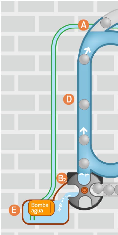
Imagen detalle salida esferas y retorno de agua al sistema
